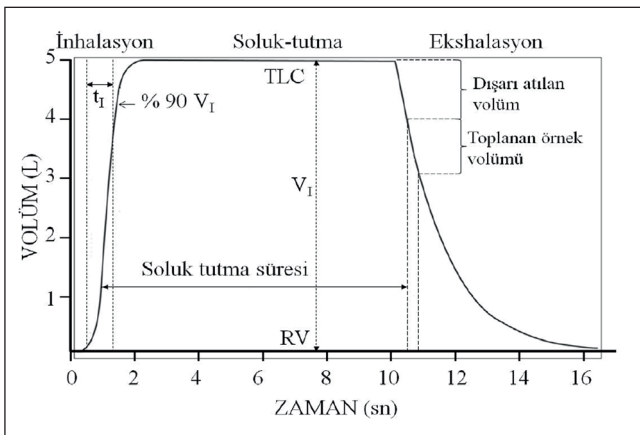
Şekil 3. Tek soluk DLCO tekniği.
